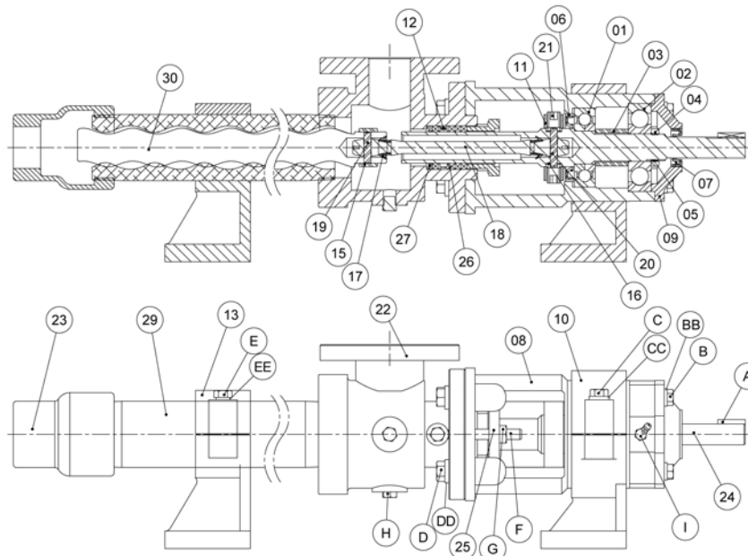
LISTA DE PIEZAS DEL MODELO SPL
